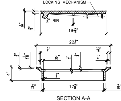
7 SECTION A-A
